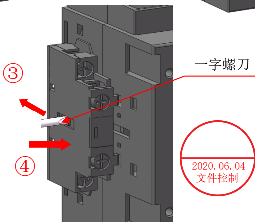
NGF1-11 安装
