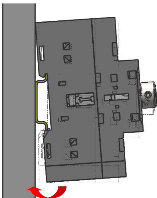
导轨安装
