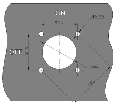
柜外 IP40 手柄操作面板开孔
