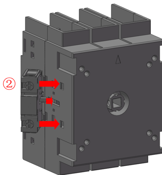
NGF1-01/10 安装
