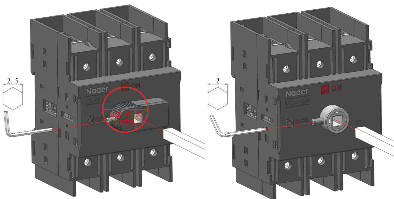
手柄轴安装
