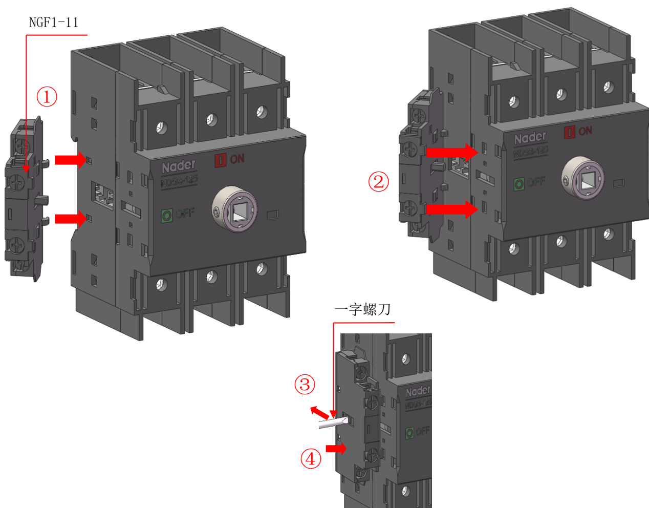
NGF1-11 安装
