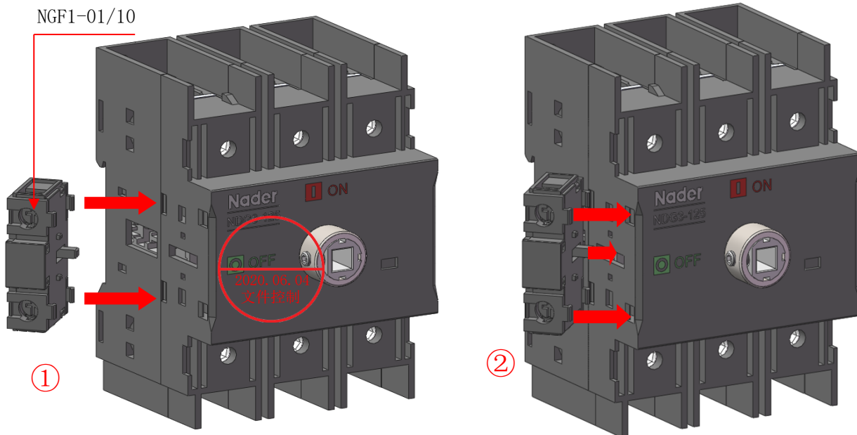
NGF1-01/10 安装
