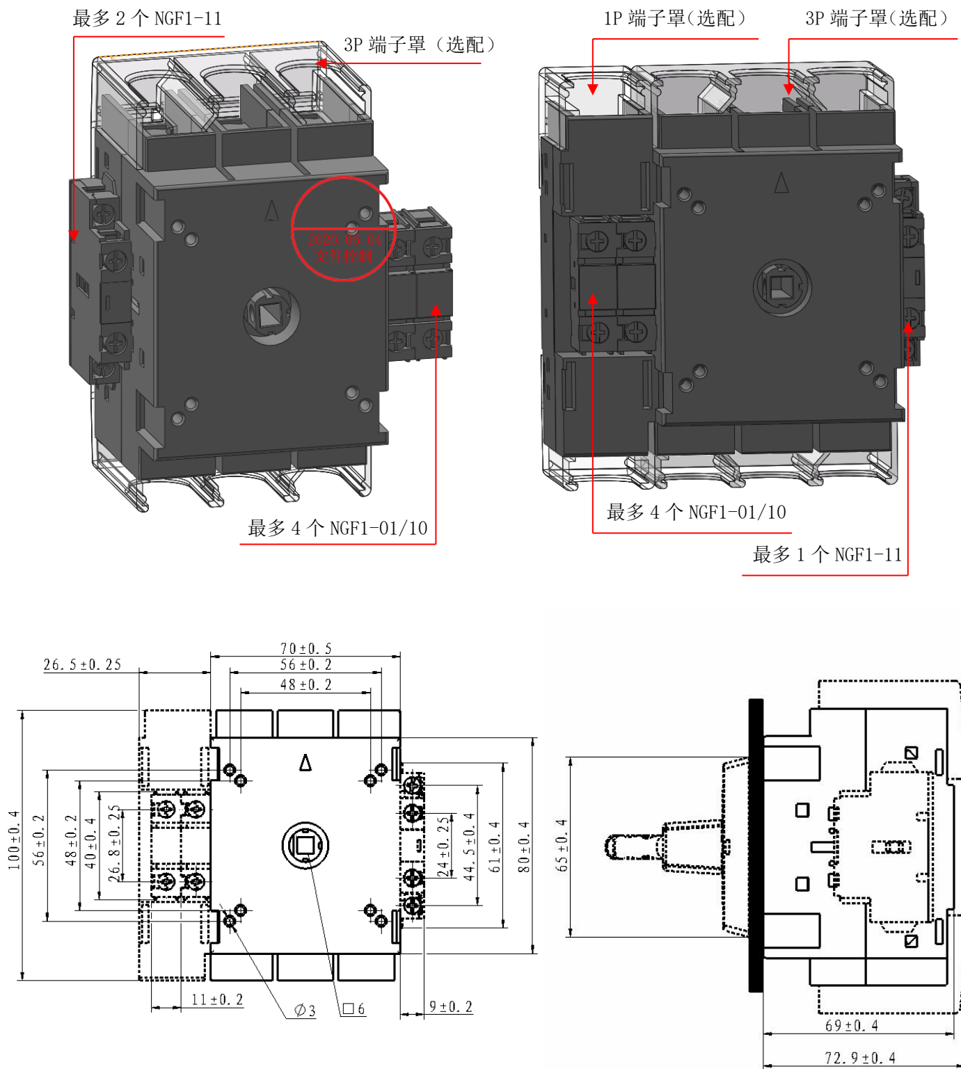
安装、外形尺寸
