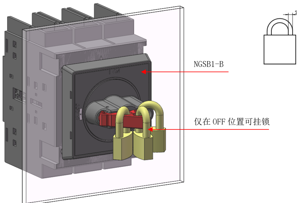
柜门安装
