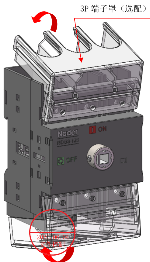
端子罩安装
