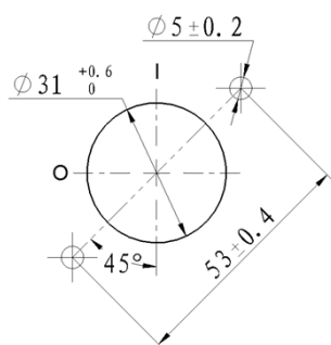
柜外 IP40 手柄操作面板开孔
