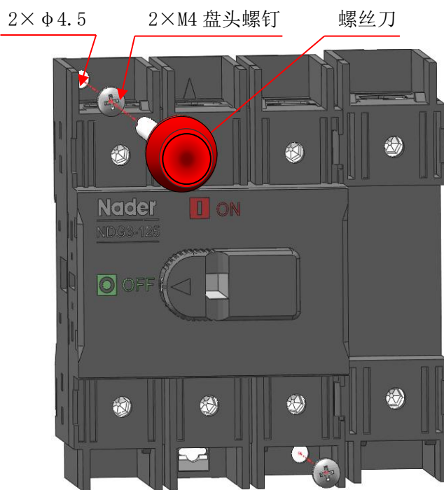
螺钉安装
