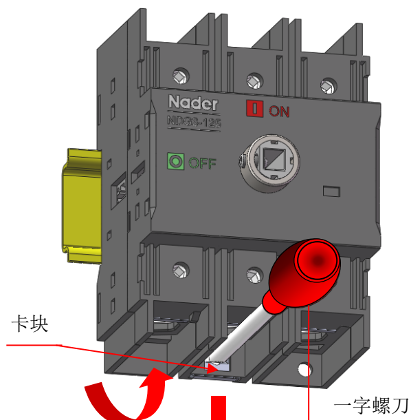
拆卸
