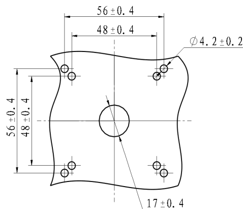
柜门安装面板开孔
